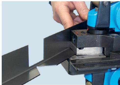
Ausklinken von rechteckigen Ausschnitten
