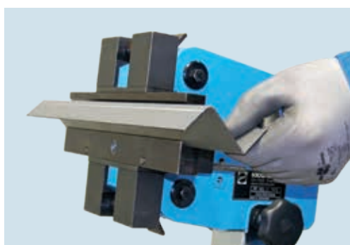
Abkanten von Blechen (nur Handformer)
