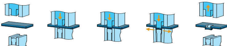
Secuencias de estados variante de clinchado S-DF
