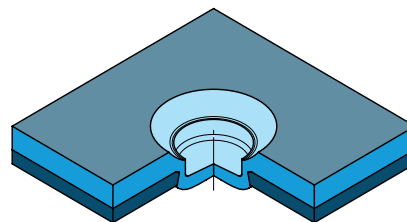
Variante de clinchado de corte por cizalla, elemento de clinchado redondo
