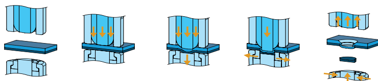
Secuencias de estados variante de clinchado de corte por cizalla
