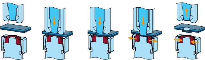
咬合连接方式 R-DF 校准顺序
