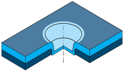
咬合连接方式 CONFIX 接合, 圆形咬合连接元件
