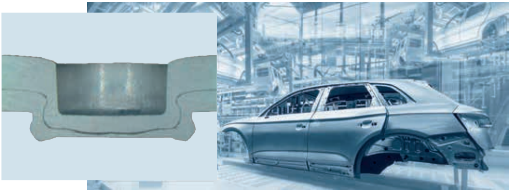
具有 R-DF-10 的最佳铆接元件
